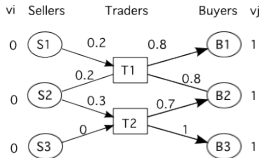
Fig.3.2 取引のネットワーク例 (b)
