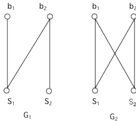
Fig.4.3 2人売手と2人買手の取引ネットワーク
