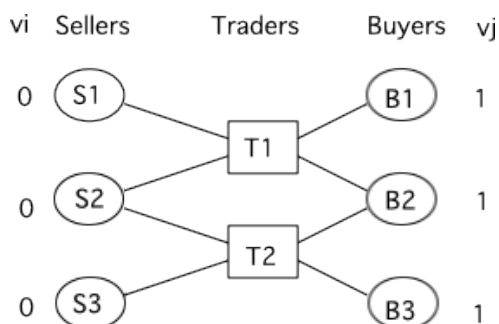
Fig.3.1 取引のネットワーク例 (a)
