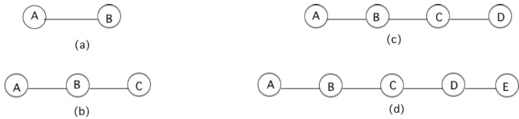
Fig.4.1 交渉ネットワークの実験
