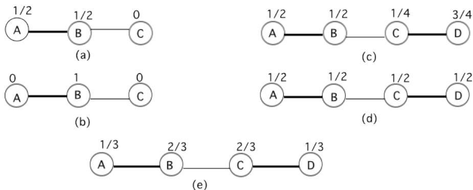
Fig.4.2 配分交渉の結果
