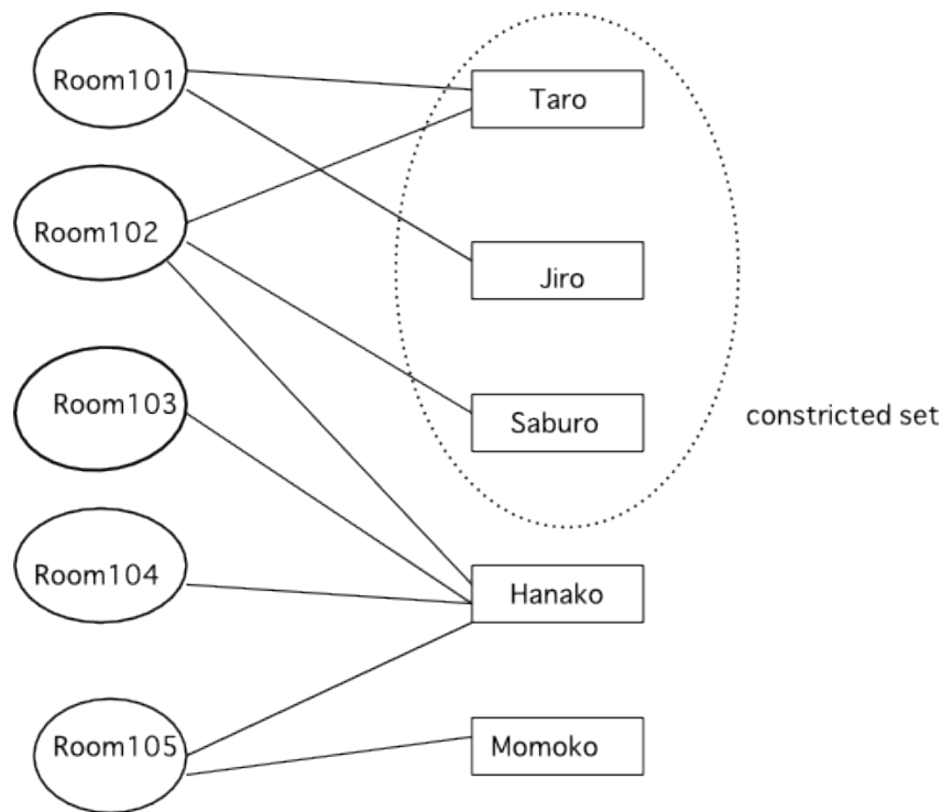
Fig.2.2 割当問題 2: 圧縮された集合
