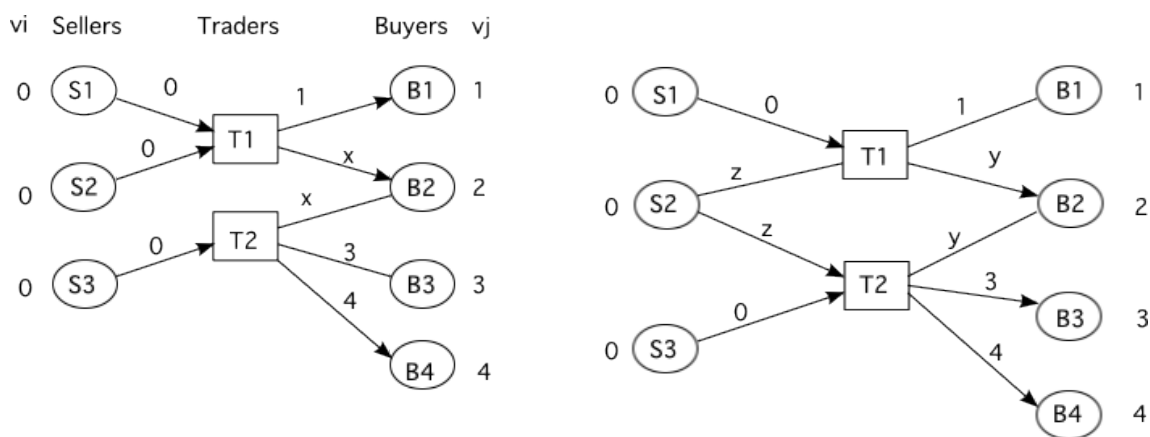
Fig.3.4 取引ネットワークにおける接続の複雑化
