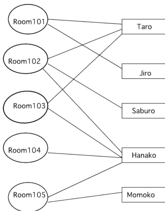
Fig.2.1 割当問題 1: 学生寮の部屋割当問題
