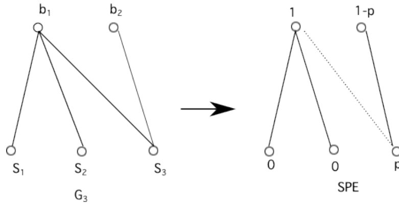
Fig.4.4 3人売手と2人買手の取引ネットワーク
